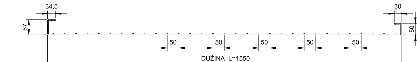
PROFIL 1:10
