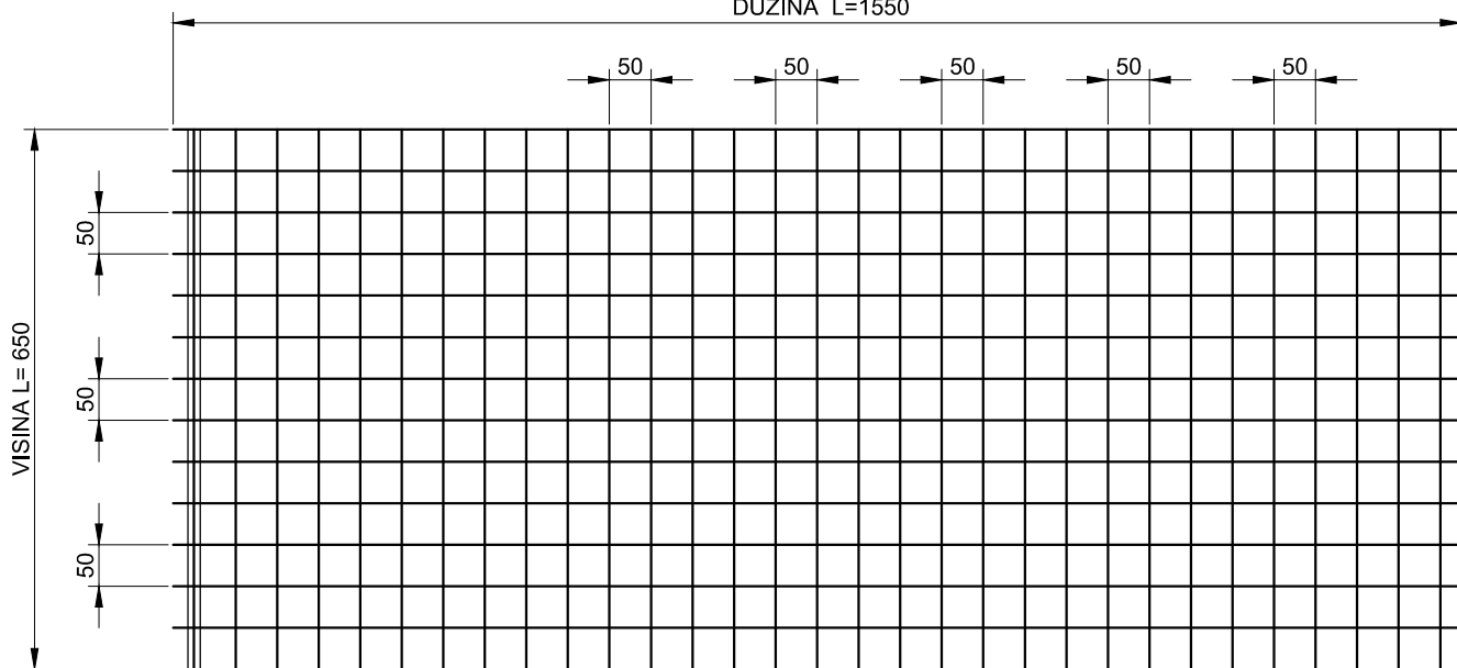
IZGLED TABLE 1:10
