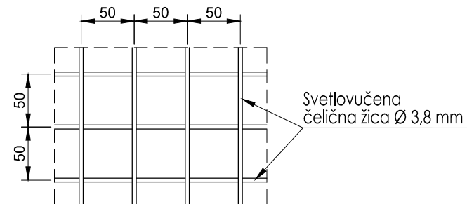
DETALJ PLETIVA 1:5
