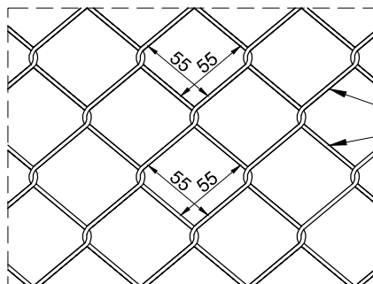
DETALJ PLETIVA 1:5
