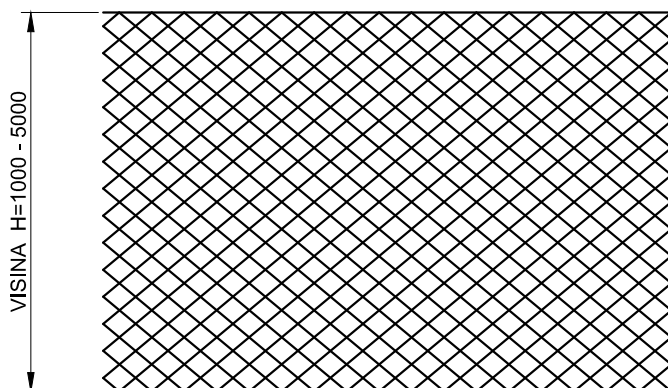
IZGLED PLETIVA 1:20
