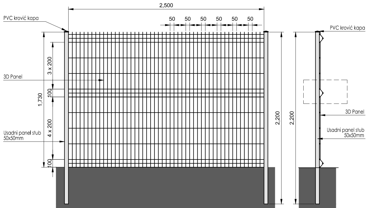
IZGLED PANELA DIMENZIJA 1730 x 2500mm R 1:25
