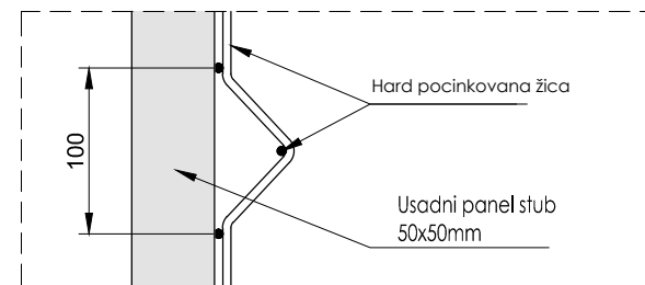
DETALJ DEFORMACIJE 1:5
